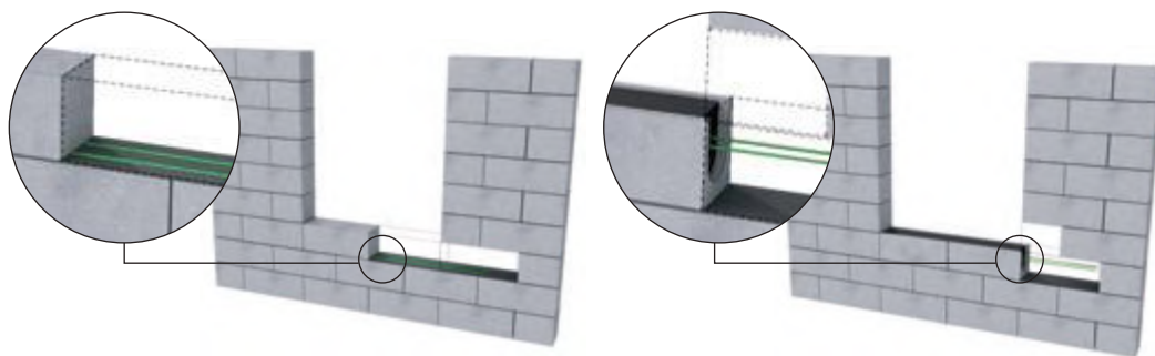
Jonction allège-trumeau porteur en maçonnerie de blocs en béton avec allège renforcée dans blocs accessoires en U
