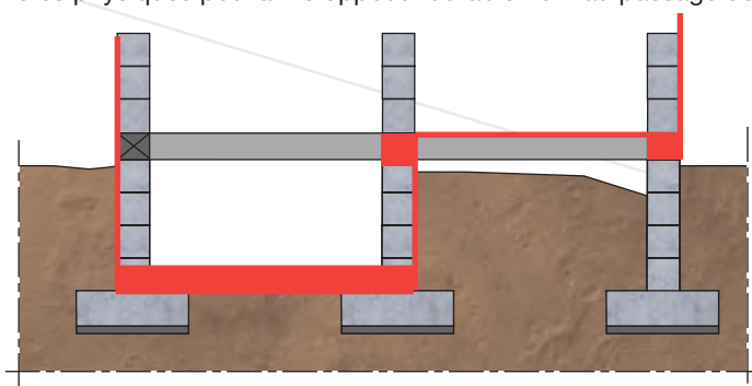
Protection contre les termites – Schéma de principe avec barrière continue
