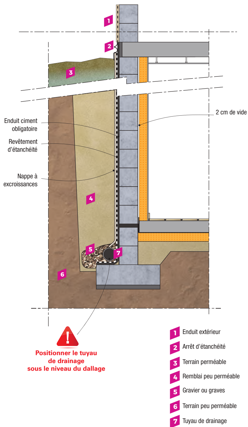
Exemple de protection d'un mur de catégorie 1
